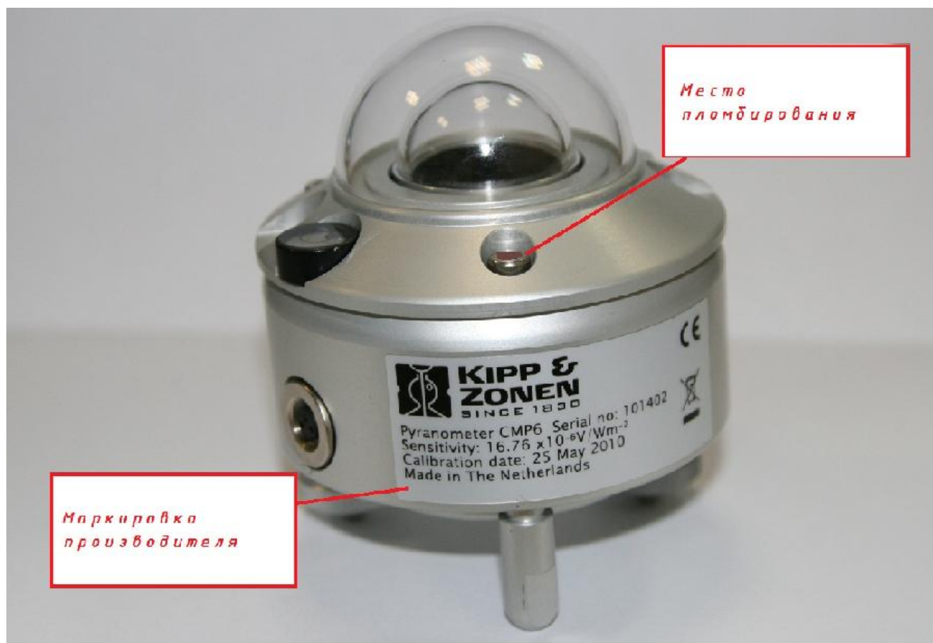
Рисунок 1 – Внешний вид пиранометра CMP6
