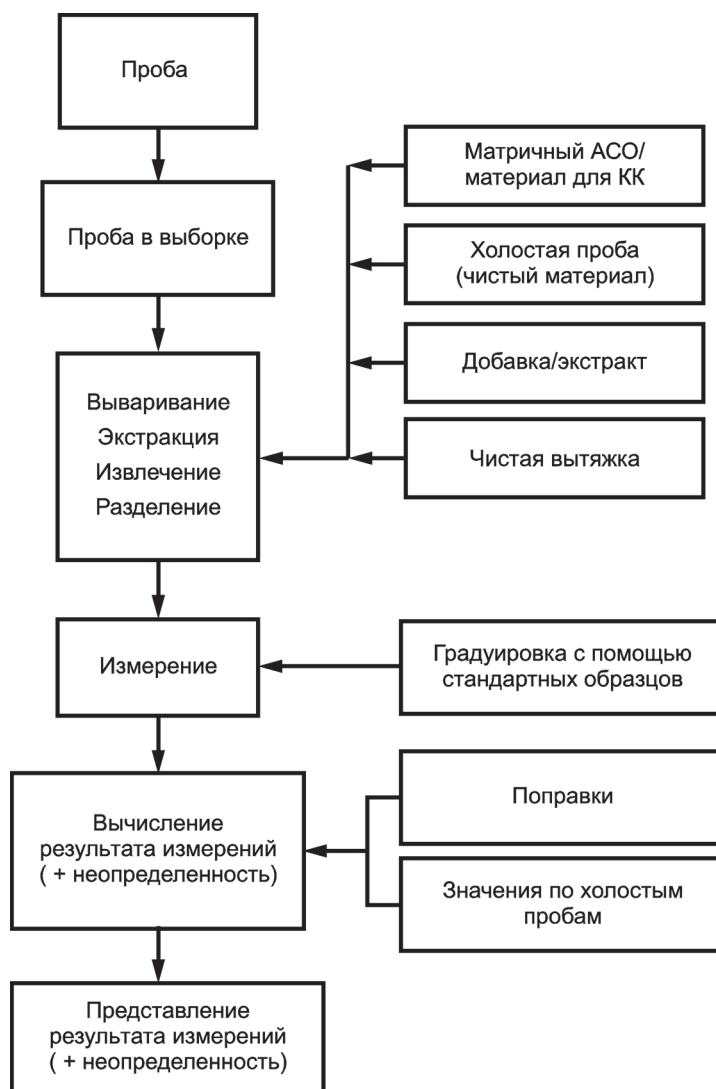
Рисунок 5 — Часть измерительной цепи
