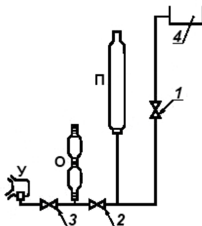
П — поверяемая пипетка; О — образцовая пипетка; У — уравнильная трубка; 1, 2, 3 — краны; 4 — резервуар для воды
