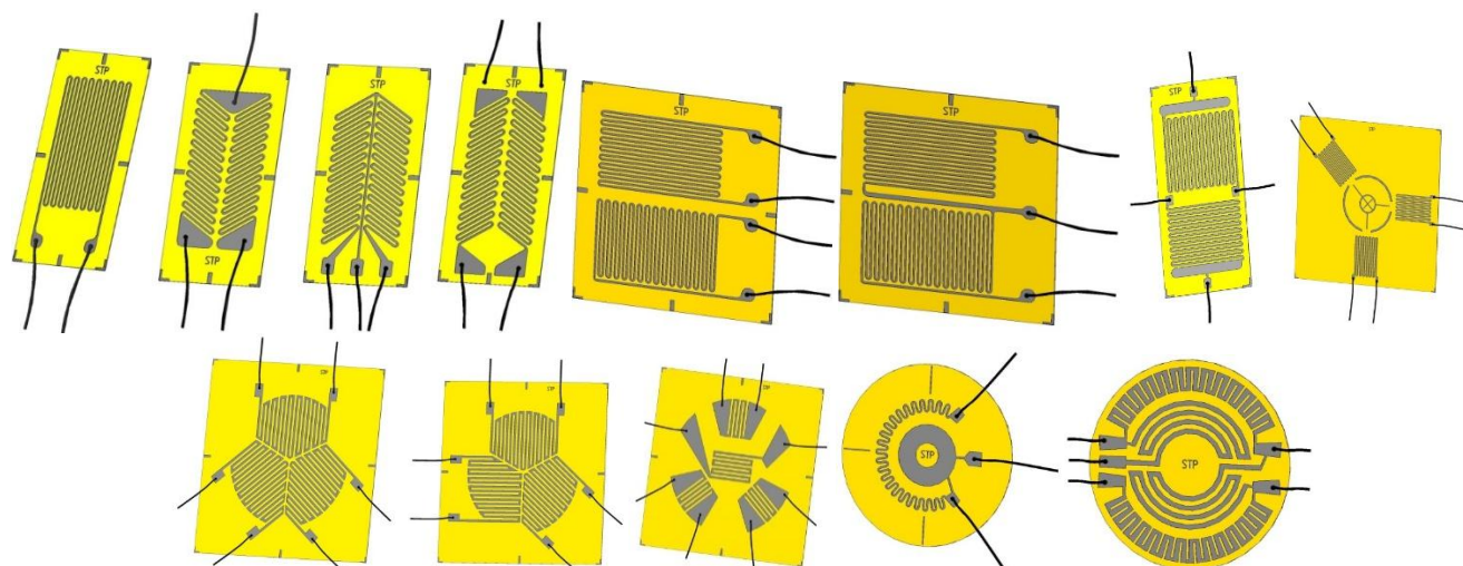
Рисунок 1 - Общий вид тензорезисторов фольговых ФК
